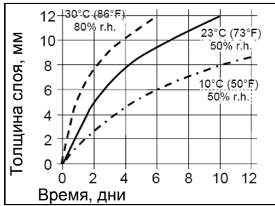
Диаграмма 1: скорость отверждения Sikaflex®-265 DG-3.
